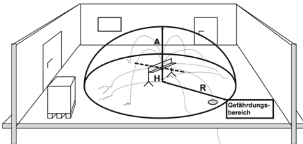
Bild 2: Gefährdungsbereich
