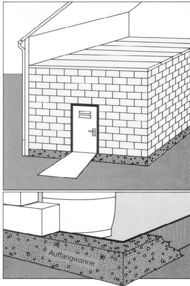
Bild 3: Musteranordnug eines Pflanzenschutzmittel-Sicherheitslagerraums
