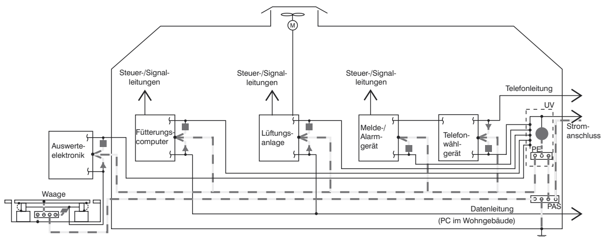
Bild 3: Überspannungsschutz für einen Schweinestall
