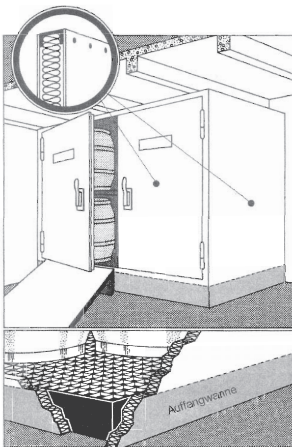
Bild 2: Muster eines Sicherheitscontainers mit Flügeltüren
