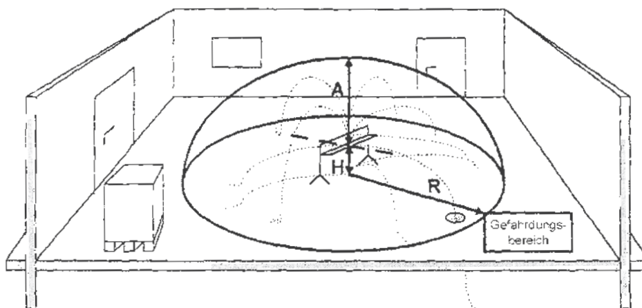
Bild 2: Gefährdungsbereich
