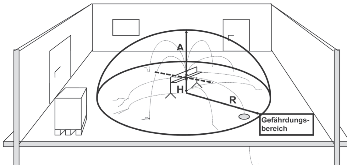
Bild 2: Gefährdungsbereich
